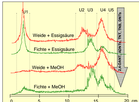
Abb. 5: Auftrennung von Wurzelextrakten mit Radio-DC
