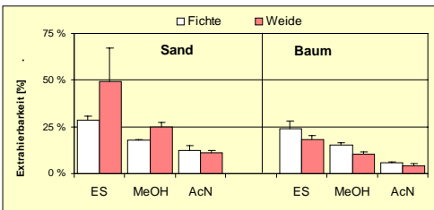
Abb. 4: Extrahierbarkeit der Radioaktivität aus Sand bzw. Bäumen von Fichte und Weide in Sandkultur
